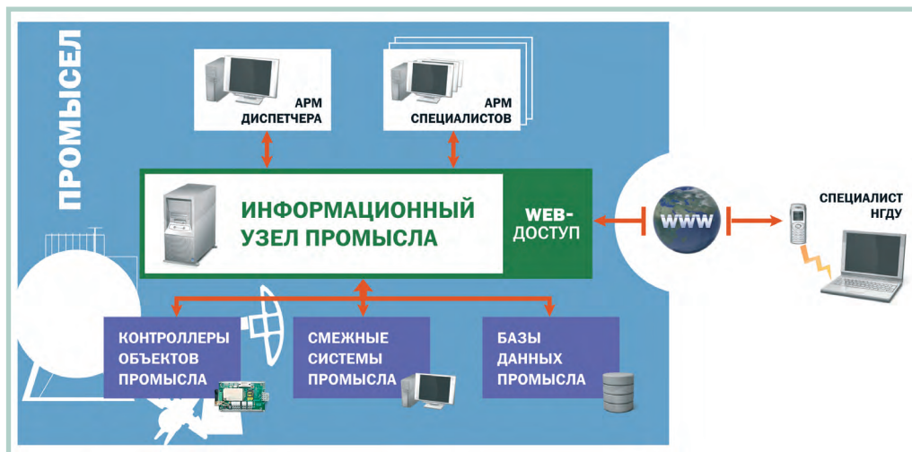
Рис. 2. Схема развёртывания системы «Мега» на промыслах
