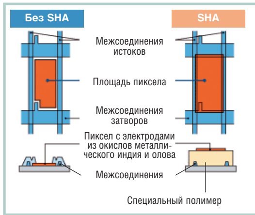
Рис. 15. Структура пиксела ЖК-дисплея, выполненного с применением технологии SHA и без неё
