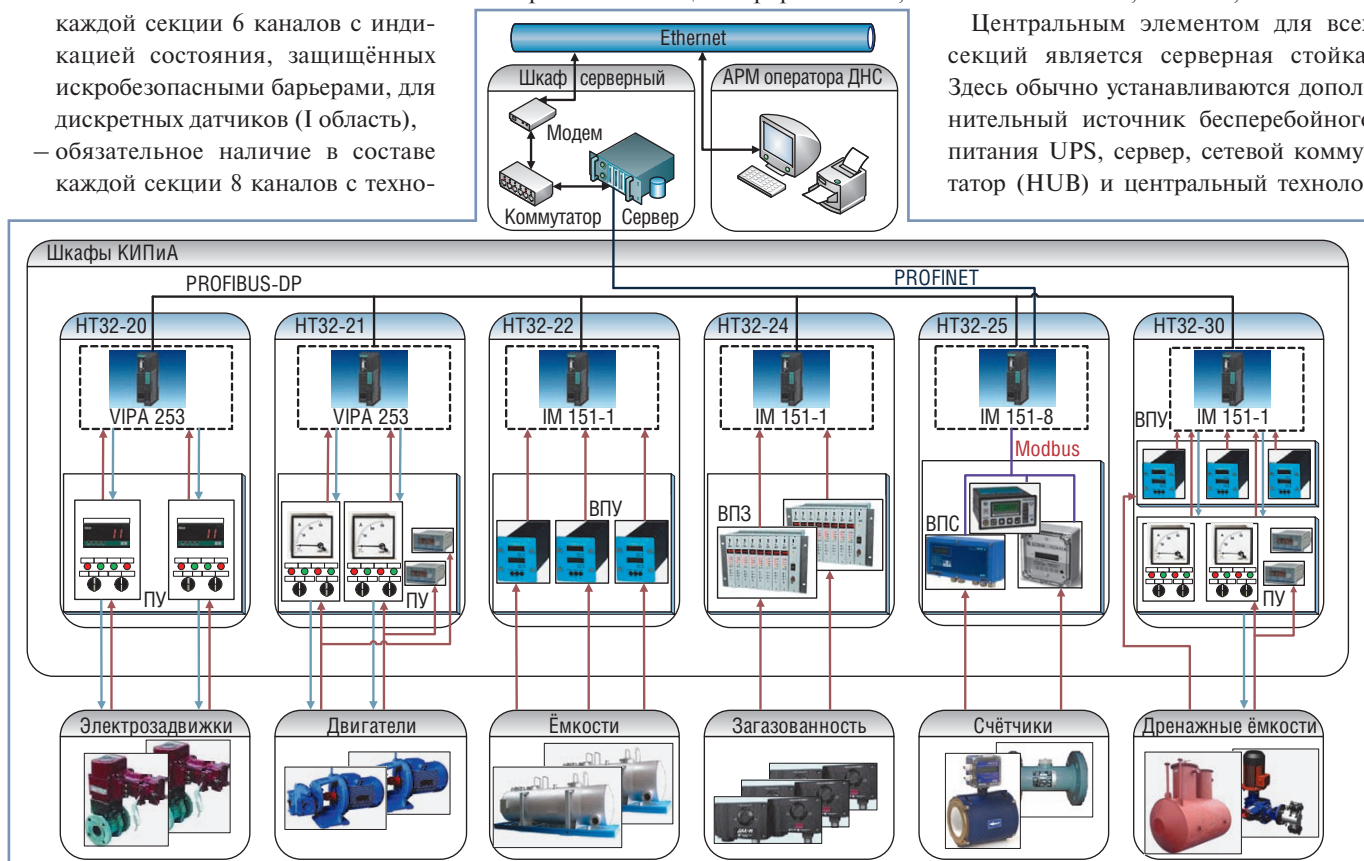
Рис. 3. Структурная схема АСУ ТП ДНС-1С Западно-Бурейкинского месторождения
