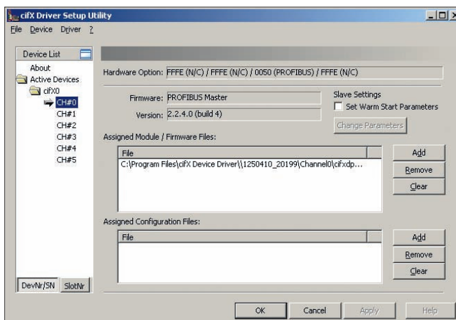
Рис. 1. Загрузка стека протокола в контроллер CIFS 50-PB
